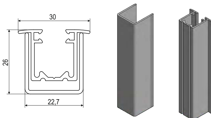
VODÍCÍ LIŠŤA ZAOMÍTACÍ S POUZDREM pro montáž k zaomítání
