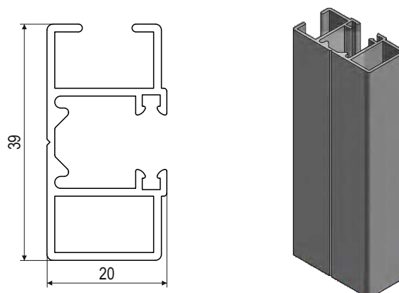
VODÍCÍ LIŠŤA PRO SAMONOSNÝ SYSTÉM STANDARD 20 x 39 mm
